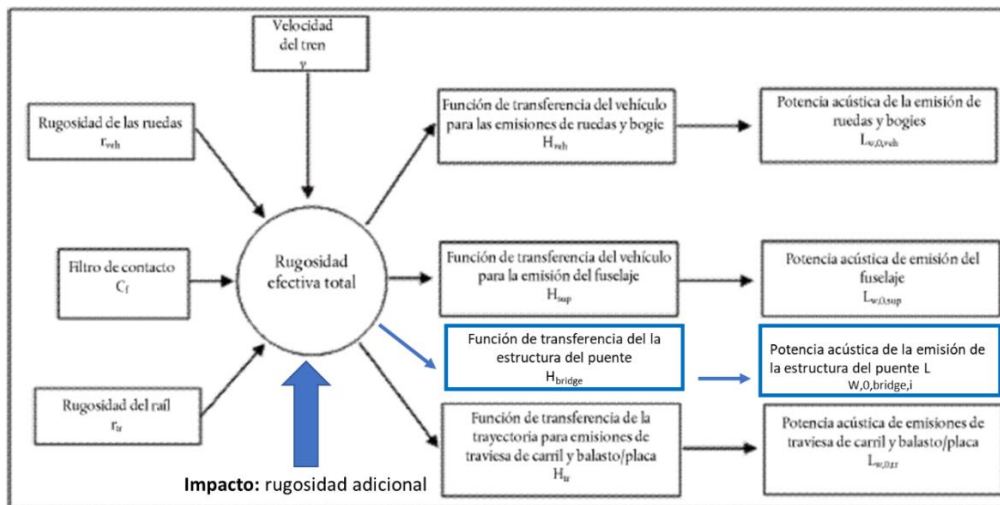
Figura 2. Esquema del concepto general del ruido de rodadura.
